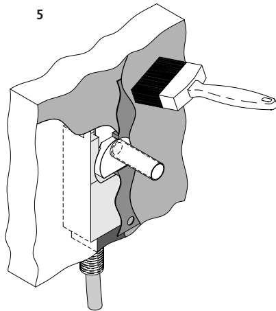
Wandbedeckung, z.B. Fliesen
