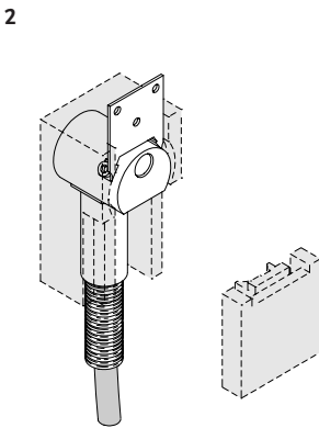
1/2"- Anschluss für Kupfer-, Kunststoff- (PEX-) oder Stahlrohre
