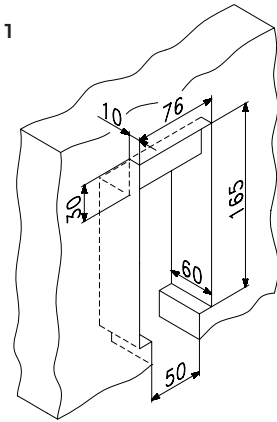
1/2"- Anschluss für Kupfer-, Kunststoff- (PEX-) oder Stahlrohre
