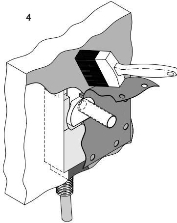
Beschichtung - 2. über Gummimembrane
