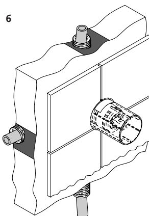
Rivestimento parete, piastrellatura
