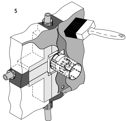
Wandbedeckung, z.B. Fliesen
