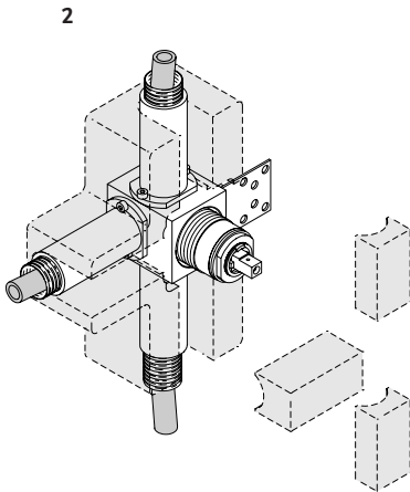
1/2"- Anschluss für Kupfer-, Kunststoff- (PEX-) oder Stahlrohre
