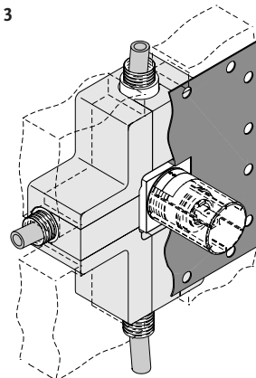
Wandangleichung
