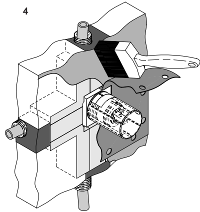
Beschichtung - 2. über Gummimembrane
