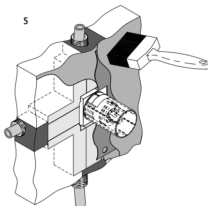
Rivestimento - La seconda mano sopra la membrana di gomma
