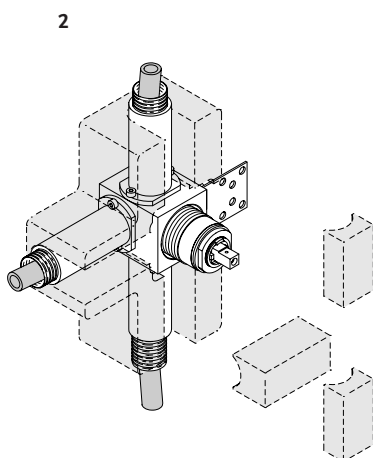
Raccordo 1/2" per tubi di rame, di plastica (tubo PEX) o di acciaio
