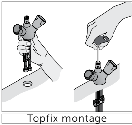
Topfix montage
