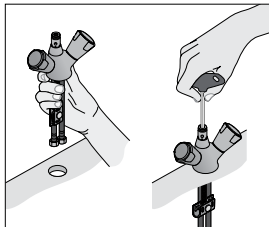
Topfix montage
